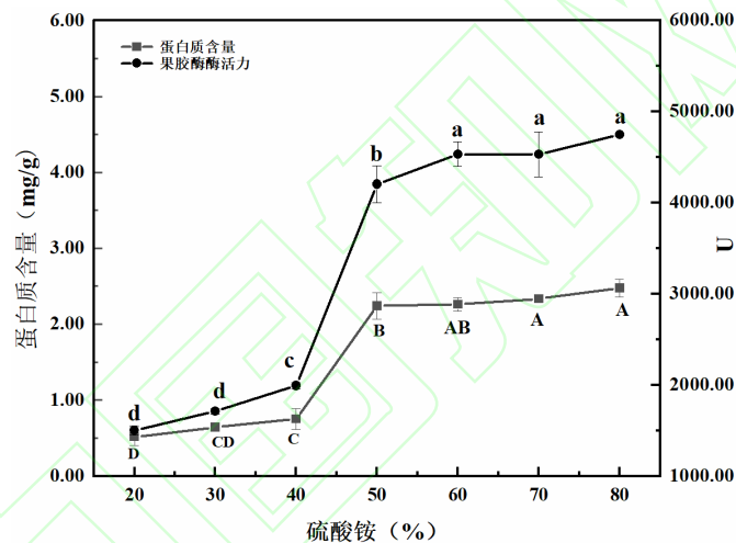
图1 硫酸铵浓度(20%~80%)对马铃薯细胞壁果胶酶粗提物酶活力及蛋白含量的影响
